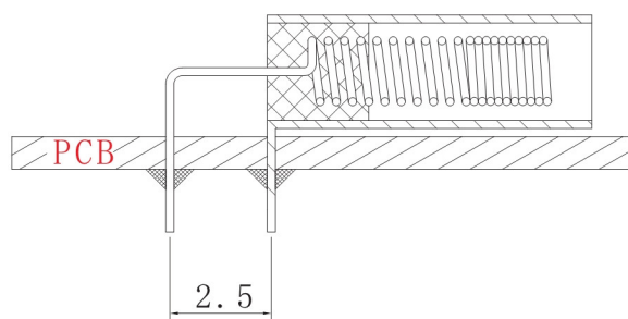
震动开关焊接位置图
