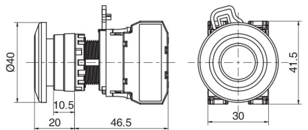
蘑菇头按钮
