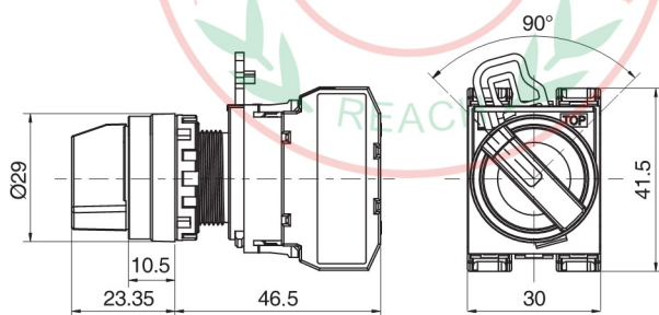
带灯选择开关2P
