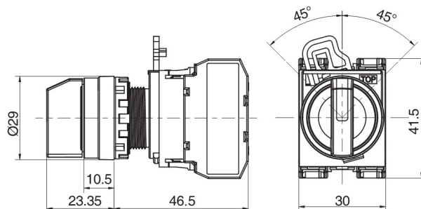
带灯选择开关3P
