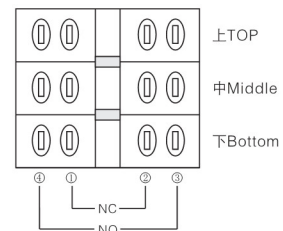
□ 端子排列图 / Terminal style
