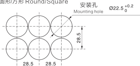
圆形/方形 Round/Square
