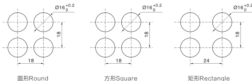
□ 安装尺寸图 / Installation size
