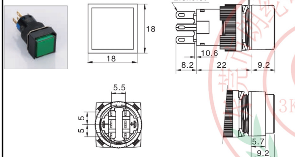
方形按钮
