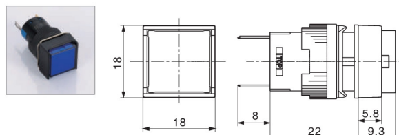
方形指示灯
