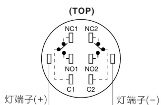
按钮开关/ Push Button
