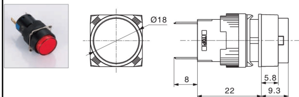
圆形指示灯
