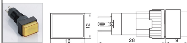
长方形指示灯/按钮
