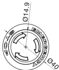
带警示灯急停按钮
