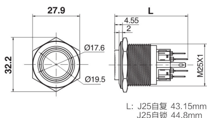
高位钮带灯
