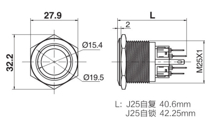
平钮带灯
