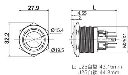
弧钮带灯
