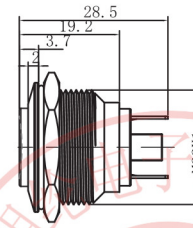
弧钮螺丝型
