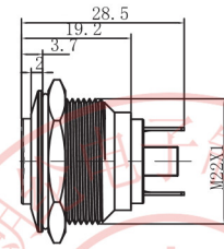
弧钮螺丝型
