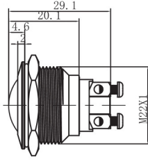
平钮螺丝型
