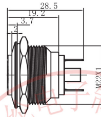
弧钮螺丝型
