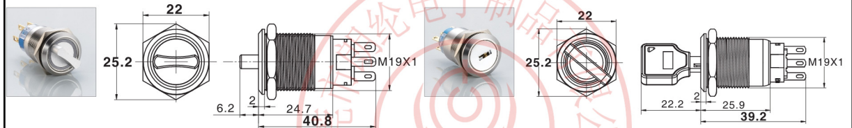
选择开关
