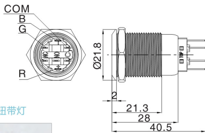
单刀/1Pole 双刀/2Pole
