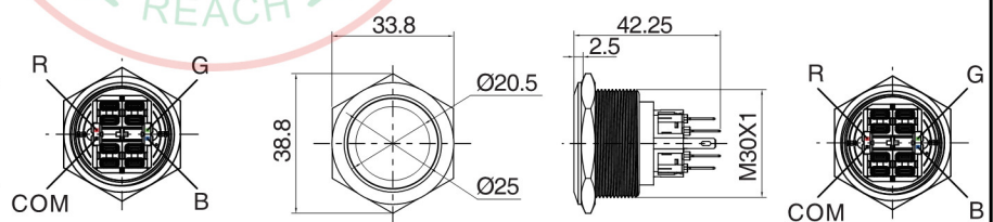
单刀/1Pole 双刀/2Pole
