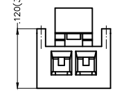
2-4Circuits
