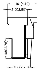
7-15Circuits
