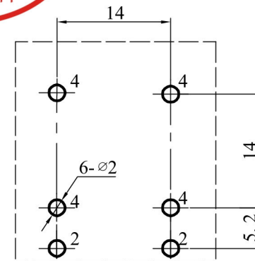
线路板
