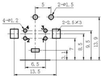
PCB板安装孔图
