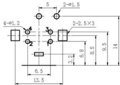
PCB板安装孔图
