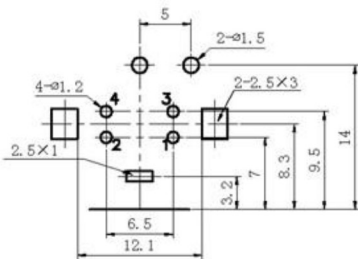
PCB板安装孔图
