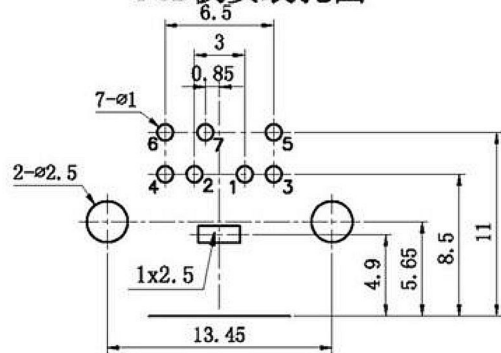
PCB板安装孔图
