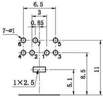
PCB板安装孔图
