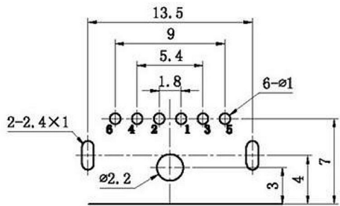
PCB板安装孔图
