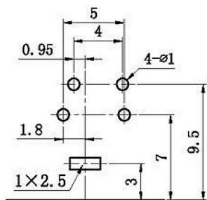
PCB板安装孔图
