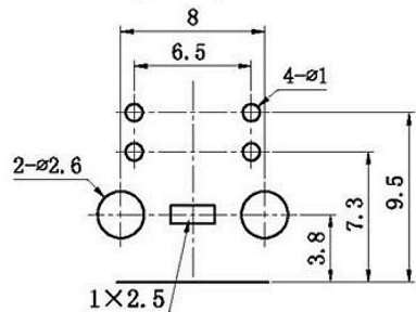
PCB板安装孔图
