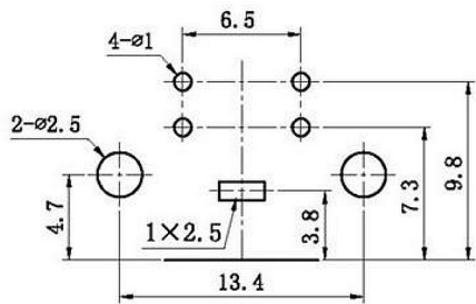
PCB板安装孔图
