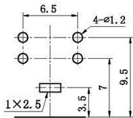
PCB板安装孔图
