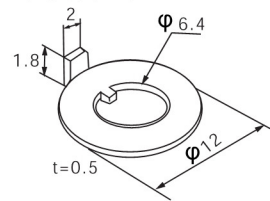
固定华司 Fix Washer
