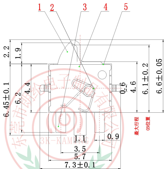
外型图 OUTLINE DRAWING
