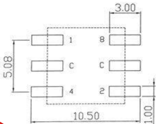
P.C.B DIMENSION
