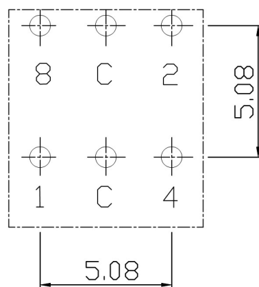
P.C.B DIMENSION
