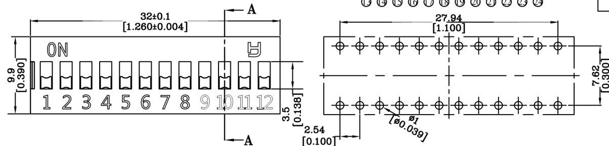
P.C.B LAYOUT
