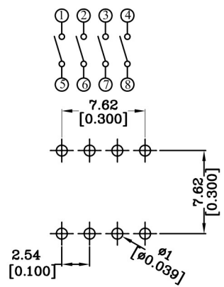
P.C.B LAYOUT
