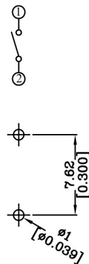
P.C.B LAYOUT
