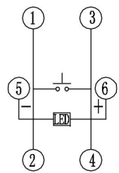
电原理图
