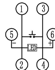
电原理图
