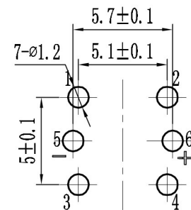
元件面孔位图
