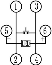
电原理图
